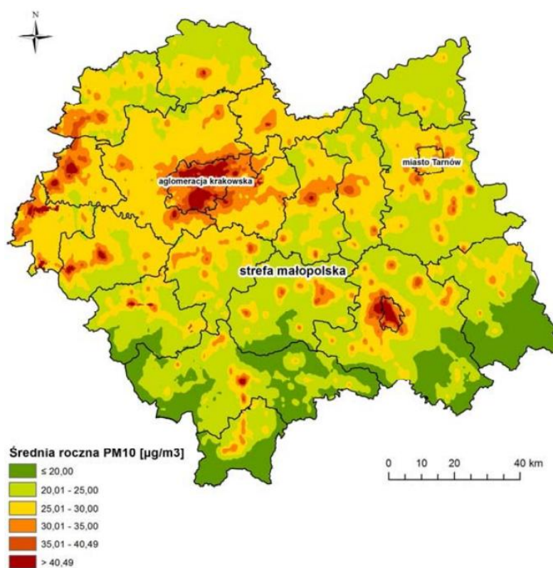
Rysunek 21. Średnioroczny rozkład stężenia PM10 [ \mu\text{g}/\text{m}^3 ]
