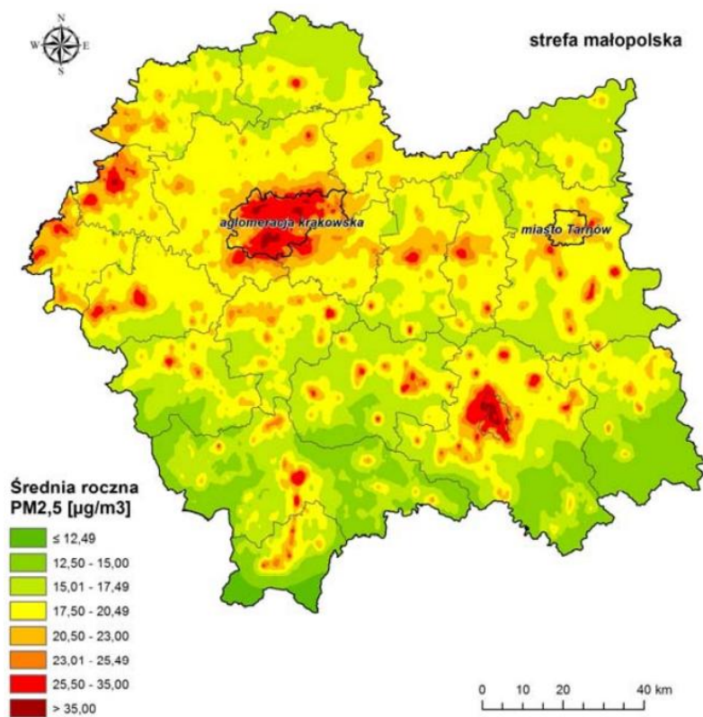
Rysunek 22. Średnioroczny rozkład stężenia PM2,5 [ \mu\text{g}/\text{m}^3 ]
