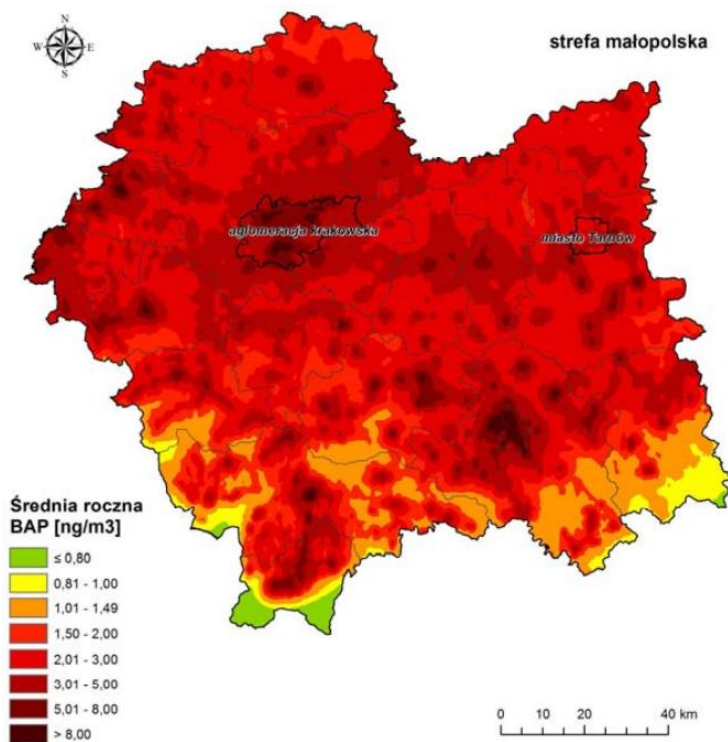
Rysunek 23. Średnioroczny rozkład stężenia benzo(α)pirenu [ \text{ng}/\text{m}^3 ]
